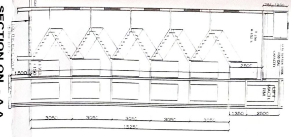
SECTION ON - A A SCALE: 1/100
